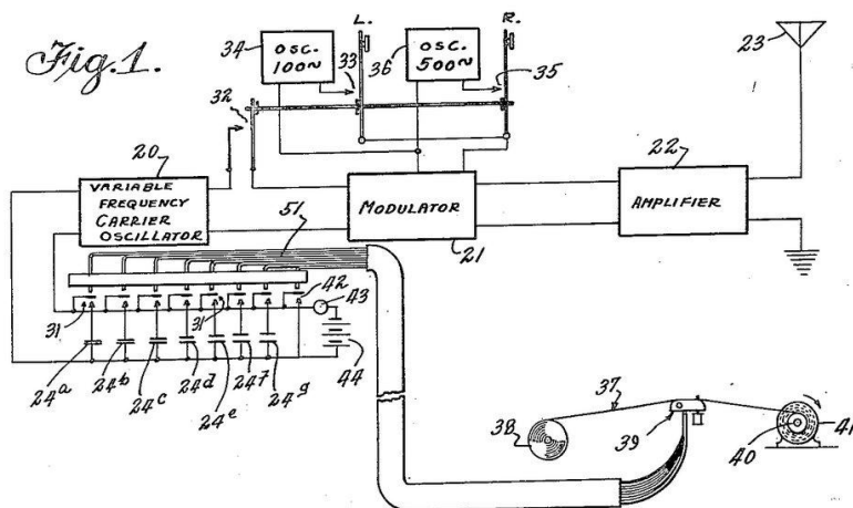
Esquema de la patente con la comunicación secreta torpedo-barco
