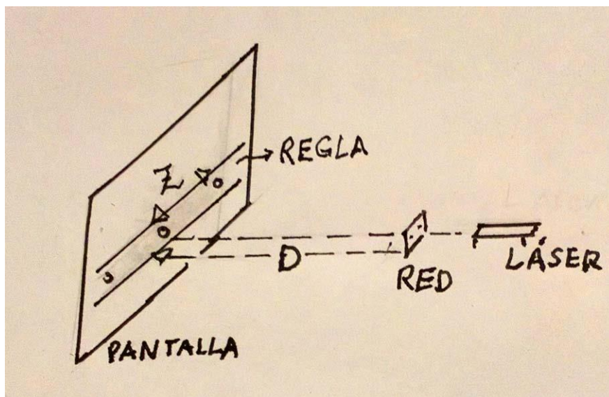
Fig.1. Esquema del dispositivo experimental. Sobre la regla aparece la mancha luminosa central y a ambos lados las manchas luminosas del primer máximo.
